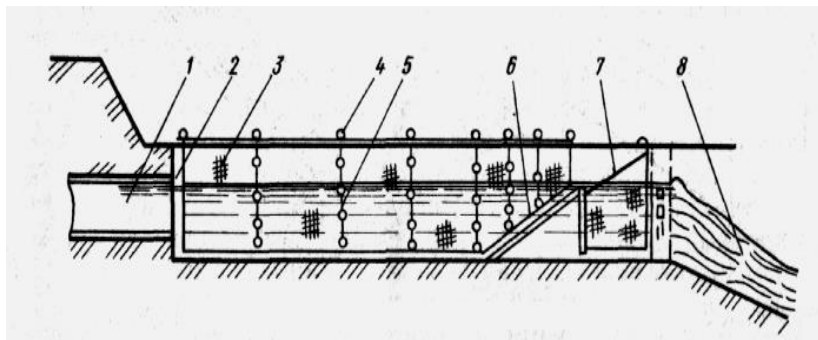
Рис. 10.2. Сетной концентратор:
