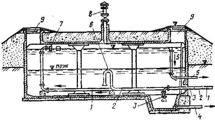
Рис. 4.18. Железобетонный резервуар:
