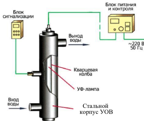
Рис. 5.7. Принципиальная схема ультрафиолетовой установки для обеззараживания воды
