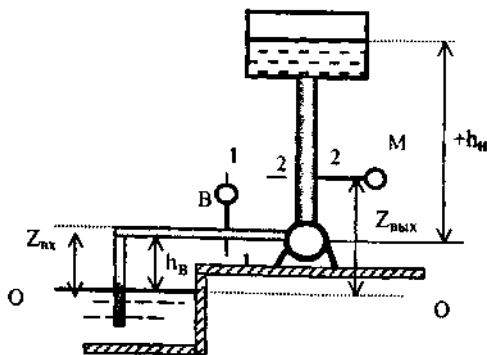
Рис. 4.6. Установка с положительными высотами всасывания и нагнетания
