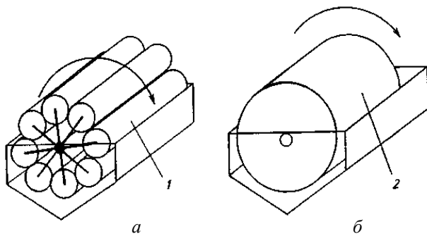
Рис. 5.16. Вращающиеся биофильтры: а – «Штеллерматик»; б – «Евроматик»; 1 – перфорированные трубы, заполненные гофрированными пластиковыми дисками; 2 – сетчатый барабан, заполненный пластиковой загрузкой
