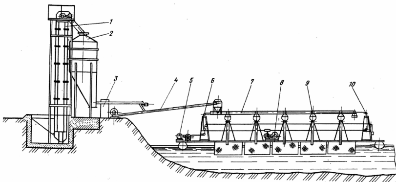
Рис. 7.17. Механизированная линия кормления: 1 – нория НЦГ-10; 2 – бункер-хранилище; 3 – пульт управления;
