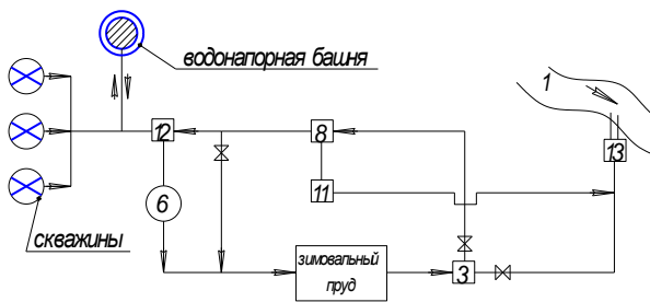
Рис. 3.4. Схема водоснабжения с забором воды из подземного водоисточника – комбинированная: 1 – водоисточник; 2 – скважины; 3 – насосная станция первого подъема; 6 – оксигенатор; 8 – сооружения для грубой очистки воды; 11 – бассейны (отстойники); 12 – сооружения для обезжелезивания, умягчения воды либо удаления углекислоты; 13 – водовыпуск
