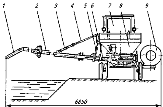
Рис. 7.3. Кормораздатчик ПД-0,6:
