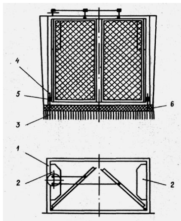
Рис. 8.13. Плавающий модуль: 1 – рама; 2 – блоки плавучести; 3 – сетка; 4 – пальцы; 5 – втулки, 6 – перфорированный материал
