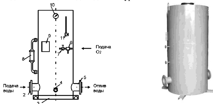
Рис. 6.2. Оксигенатор:
