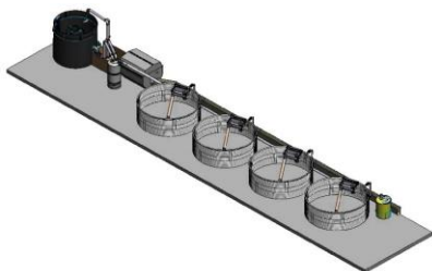
Рис. 2.2. Модуль типа «FTPE 10» для выращивания рыбы в условиях УЗВ
