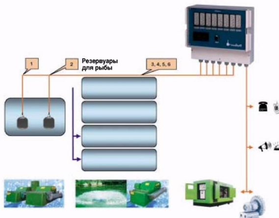
Рис. 9.22. Система «Oxy Guard-Commander»
