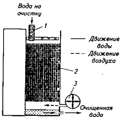
Рис. 5.14. Орошаемый биофильтр: 1 – реактивный ороситель; 2 – загрузка; 3 – воздушный насос
