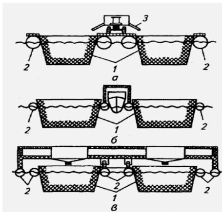
Рис. 10.12. Схема различных типов плавучих садковых хозяйств: 1 – сетчатые садки; 2 – понтоны; 3 – кормораздатчики; (а – тракторный; б – плавучий или лодочный; в – плавучий на кран-балке)
