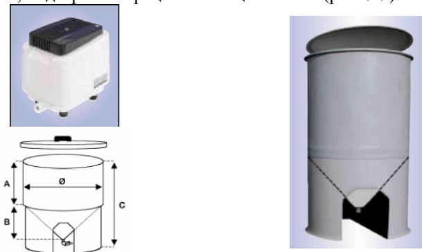
Рис. 9.9. ART-емкости для зоопланктона и артемий
