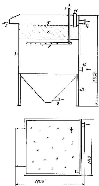
Рис. 5.5. Комбинированный фильтр КФ-10:
