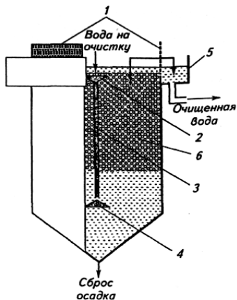
Рис. 5.15. Биофильтр с регенерируемой загрузкой из полиэтиленовых гранул: 1 – сетка; 2 – приемная воронка; 3 – гидроэлеватор; 4 – отбойная тарелка; 5 – водосборное кольцо; 6 – загрузка (полиэтиленовые гранулы диаметром 2,5 мм)
