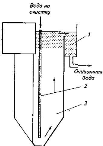
Рис. 5.13. Биофильтр с песчаной загрузкой: 1 – водосборное кольцо; 2 – водоподводящая труба; 3 – загрузка (песок, удерживаемый во взвешенном состоянии током воды)
