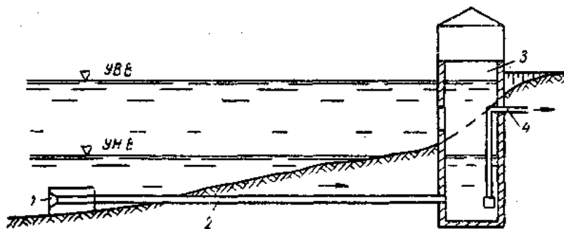
Рис. 3.7. Водоприемник руслового типа: 1 – оголовок; 2 – самотечные трубы; 3 – береговой колодец; 4 – к насосам
