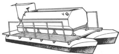
Рис. 7.1. Кормораздатчик СКР-1,5
