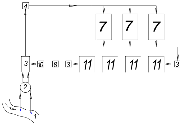
Рис. 3.3. Замкнутая напорная схема водоснабжения: 1 – водоисточник; 2 – водозабор; 3 – насосная станция первого подъема; 4 – сооружение для обеззараживания воды; 7 – рыбоводные бассейны (пруды); 8 – сооружения для грубой очистки воды; 10 – сооружения для тонкой очистки воды; 11 – бассейны (отстойники)
