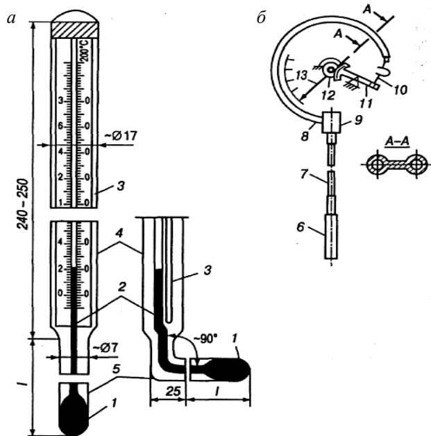
Рис. 5.17. Термометры расширения: a – технический жидкостный стеклянный; б – показывающий манометрический
