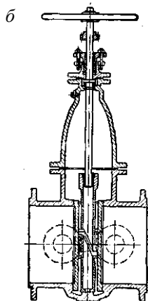
Рис. 4.13. Параллельная задвижка: а – с выдвигаемым шпинделем; б – с неподвижным шпинделем
