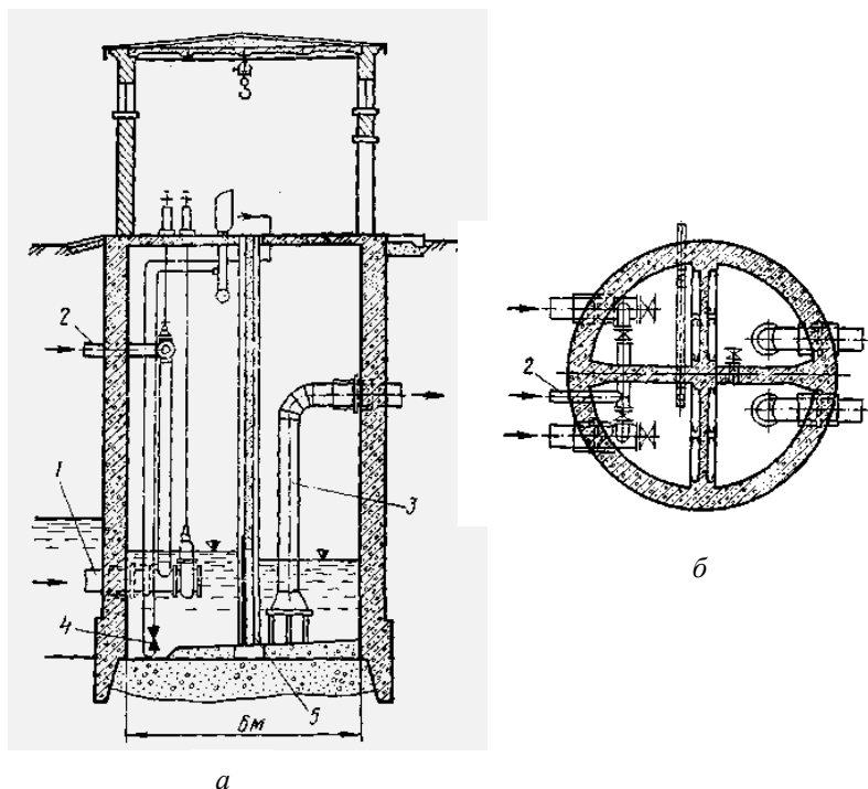
Рис. 3.9. Приемно-сеточный колодец: a – разрез; б – план; 1 – самотечные трубы; 2 – промывные трубы; 3 – всасывающие трубы; 4 – водоструйный насос (гидроэлеватор); 5 – сетки; 6, 7 – задвижки
