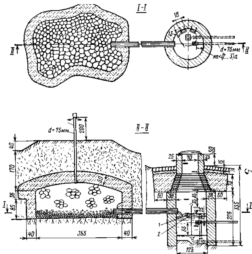
Рис. 3.12. Простейший каптаж восходящего источника с каменной наброской: 1 – рабочий уровень; 2 – предельно наивысший уровень
