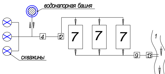
Рис. 3.5. Схема водоснабжения самотечная-прямоточная с забором воды из подземного водоисточника: 1 – водоисточник; 2 – скважины; 4 – сооружения для обеззараживания воды; 7 – рыбоводные бассейны (пруды); 9 – сооружения биологической очистки воды; 12 – сооружения для обезжелезивания, умягчения воды либо удаления углекислоты; 13 – водовыпуск
