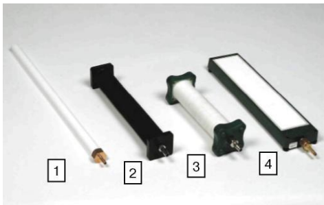
Рис. 6.12. Диффузоры:
