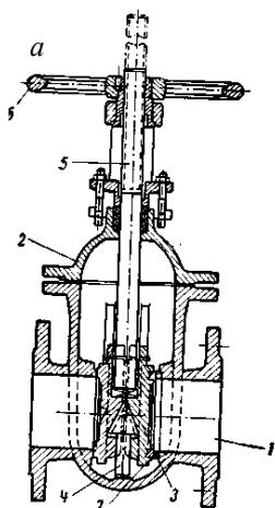
Рис. 4.13. Параллельная задвижка: а – с выдвигаемым шпинделем; б – с неподвижным шпинделем
