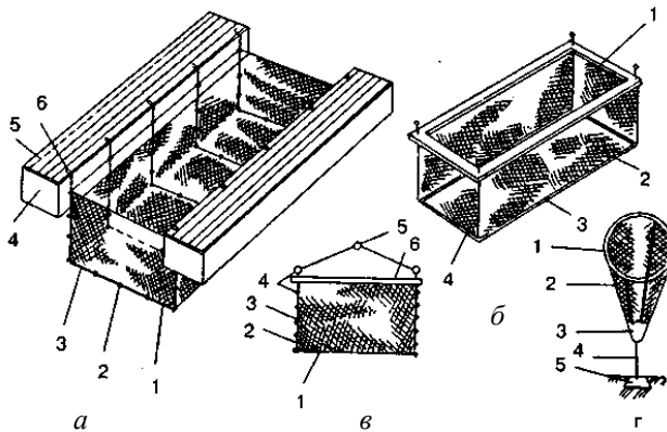
Рис. 10.7. Садки: а – гибкий: 1 – торцевая стенка; 2 – направляющие стяжные кольца; 3 – стяжной фал; 4 – понтон; 5 – настил; б – концы стяжных фалов; б – полужесткий с нижней рамкой: 1 – верхняя рама; 2 – боковая стенка; 3 – нижняя кольцевая рама; 4 – угловой фал для подъема нижней рамы; в – полужесткий с угловыми стержнями: 1 – нижняя кольцевая рама; 2 – боковая стенка; 3 – направляющие кольца; 4 – угловые стержни; 5 – кольцо для подъема; б – рама; г – конусный каркасный: 1 – жесткий каркас; 2 – стенка садка; 3 – парусиновое дно; 4 – талреп; 5 – якорь
