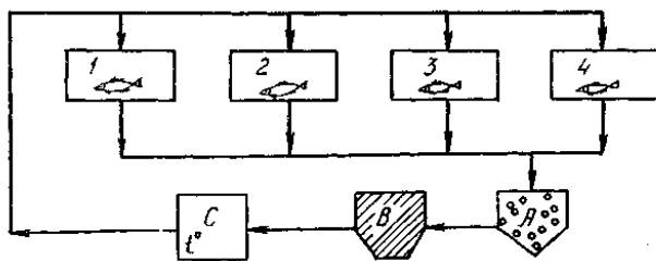
Рис. 5.9. Схема очистки воды с использованием аэротенка:
