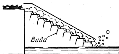
Рис. 6.9. Решетчатый аэратор
