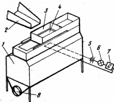
Рис. 8.1. Контейнер с весоизмерителем: 1 – контейнер; 2 – лоток от рыбоперегрузателя; 3 – передвижной двухсекционный короб; 4 – платформа весов; 5 – батарейка питания; 6 – сигнальная лампа; 7 – счетчик; 8 – слив
