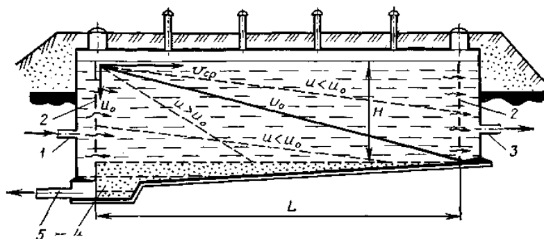
Рис. 5.1. Схема горизонтального отстойника:
