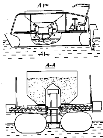
Рис. 7.2. Кормораздатчик КРБ-2
