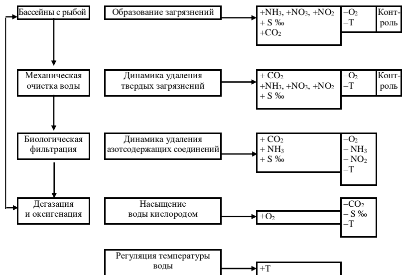
Рис. 2.1. Изменение параметров рыбоводных систем и оценка их качества
