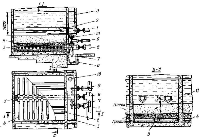
Рис. 5.4. Скорый фильтр:
