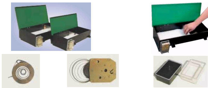
Рис. 7.10. Автоматические кормушки с часовым механизмом
