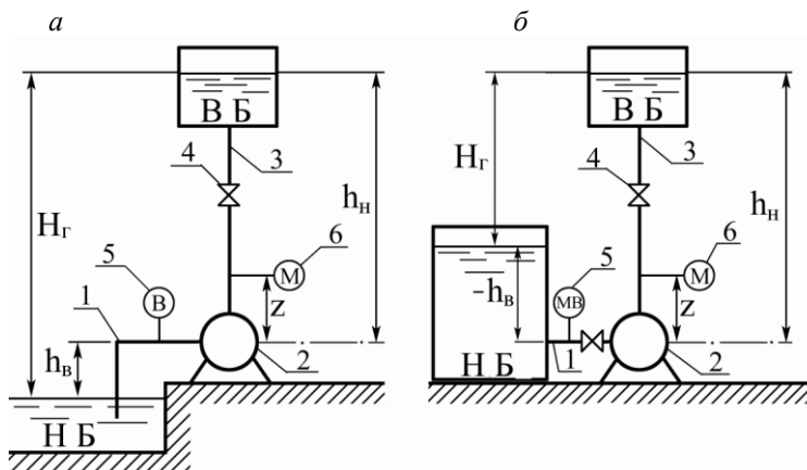
Рис. 4.4. Схемы насосной установки: а – с положительной высотой всасывания; б – с отрицательной высотой всасывания
