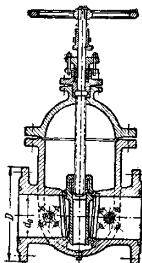
Рис. 4.14. Клиновая задвижка с неподвижным шпинделем
