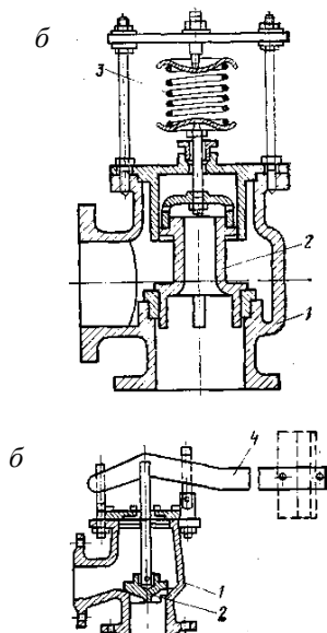
Рис. 4.17. Предохранительные клапаны: а – пружинный; б – рычажно-грузовой; 1 – корпус; 2 – клапан; 3 – пружина; 4 – рычаг
